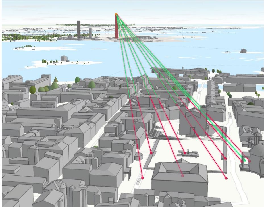
Bild 31. Siktlinjer från tornets högsta punkt till valda punkter på och intill Stortorget.
