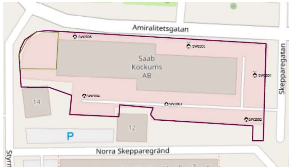
Bild 45. Placering av provgropar och grundvattenrör på fastigheten Pollux 32.
