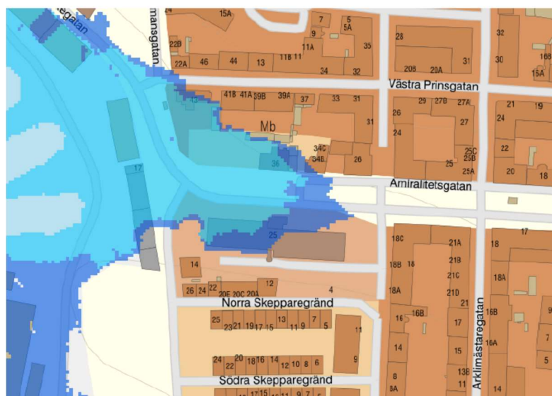
Bild 49. Stigande havsvattennivåer, 3 meter.
