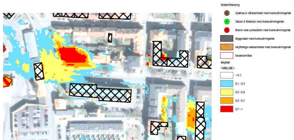
Bild 48. Utdrag ur skyfallskarteringen från 2017.
