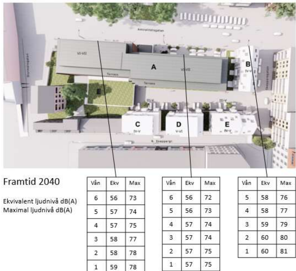
Bild 44. Ekvivalent och maximal ljudnivå dB(A) redovisat per våningsplan för år 2040.
