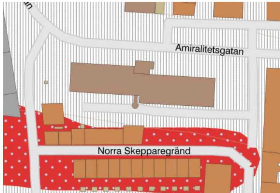
Bild 35. Jordartskarta från SGU över planområdet.
