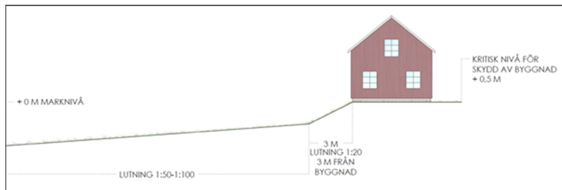
Figur 10. Princip för höjdsättning (Illustration: Norconsult)
