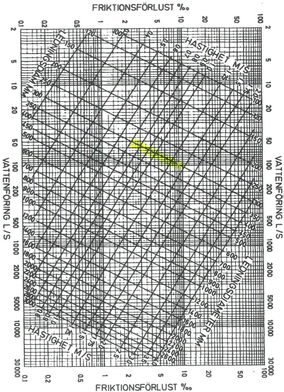
Figur 10.5 Friktionsdiagram, k = 1,0 \text{ mm} .
