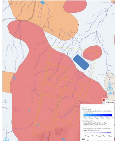
Bild 14. Utdrag ur dagvattenutredning som visar lämpligt område, blå polygon, för infiltration och fördröjning.
