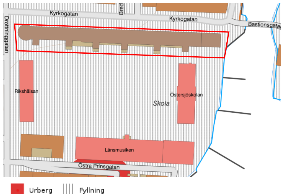
Figur 3. Översiktlig situationsbild av provtagningsområdet, mörkrött är urberg och grårandigt fyllnadsmassor. Undersökningsområdets ungefärliga läge är markerat i rött (SGU, 2024a).
