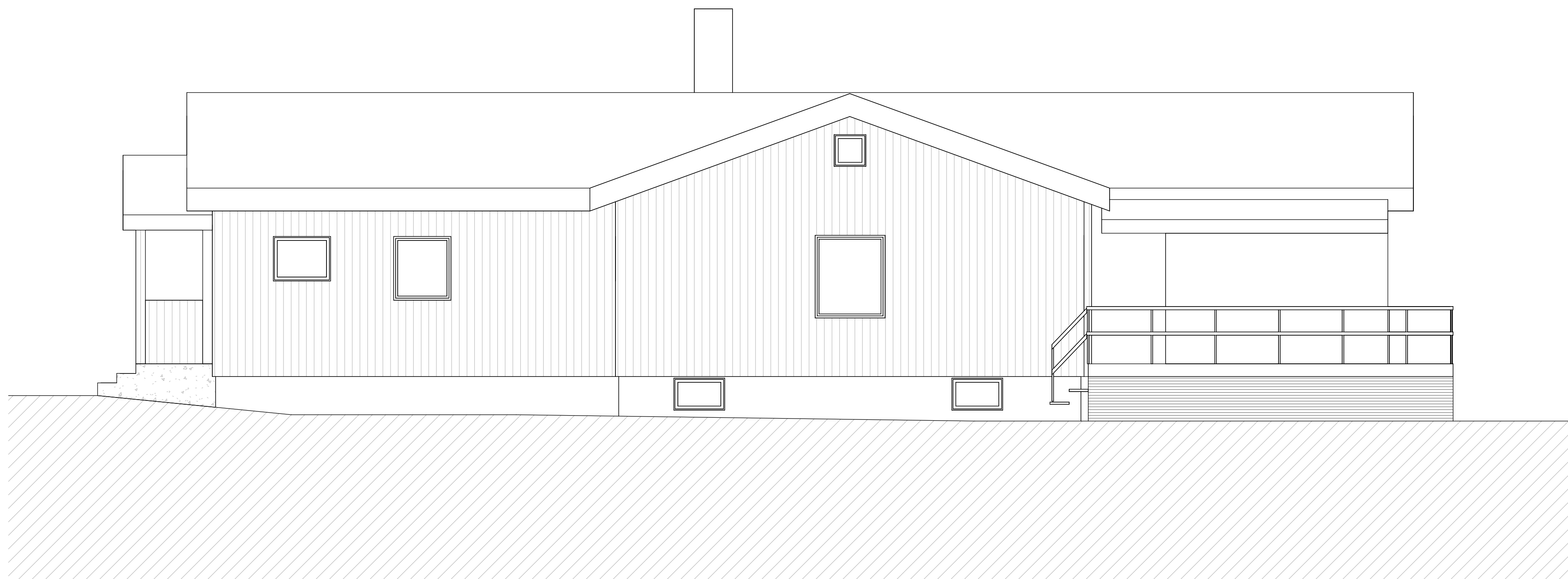
6 FASAD VÄSTER 1 : 50
