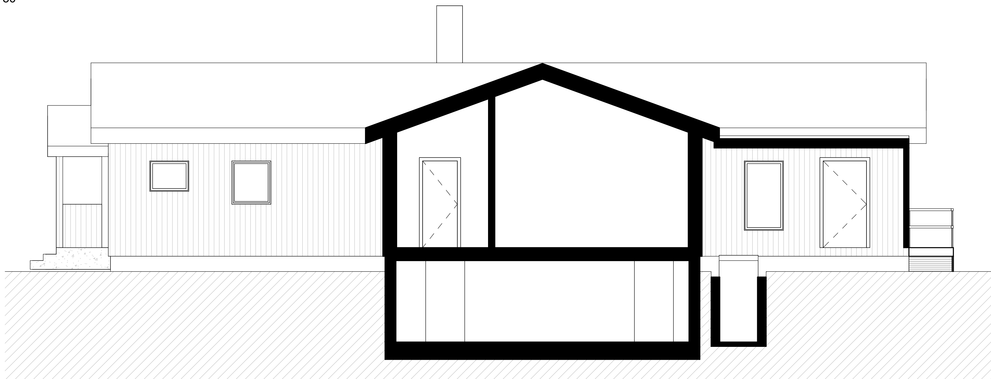
1 SEKTION A-A1 1 : 50
