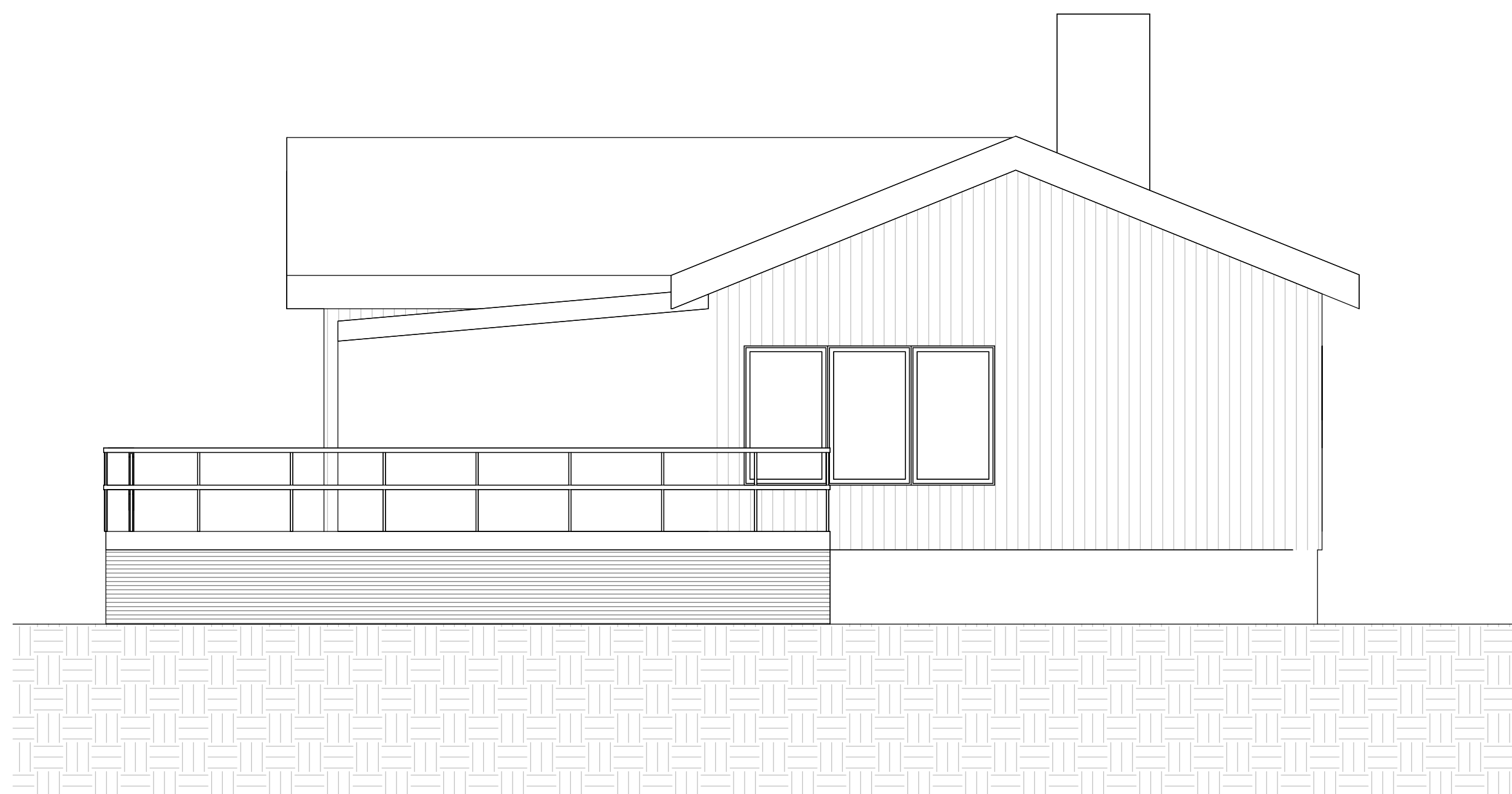
5 FASAD SÖDER 1 : 50
