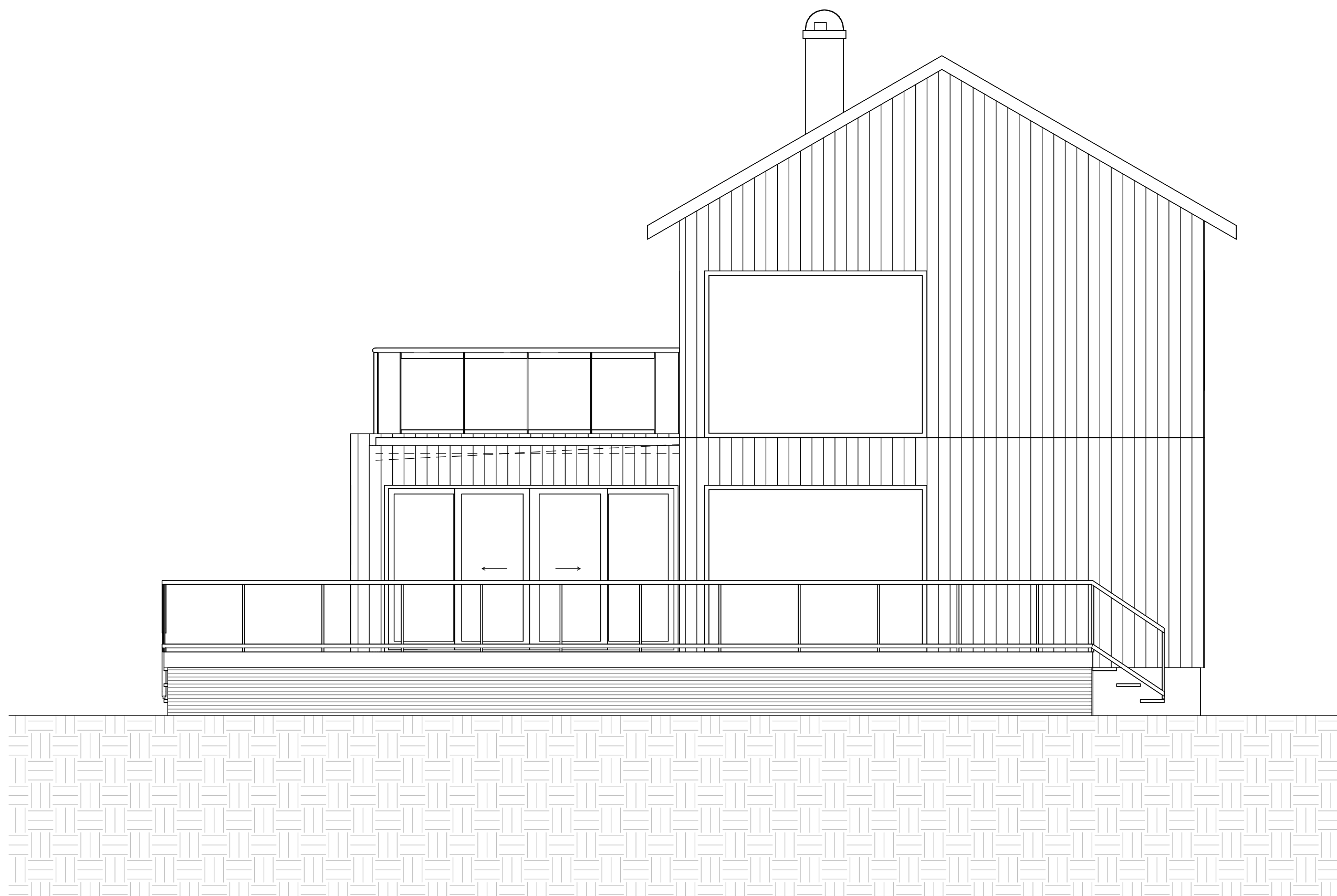
5 FASAD SÖDER 1 : 50
