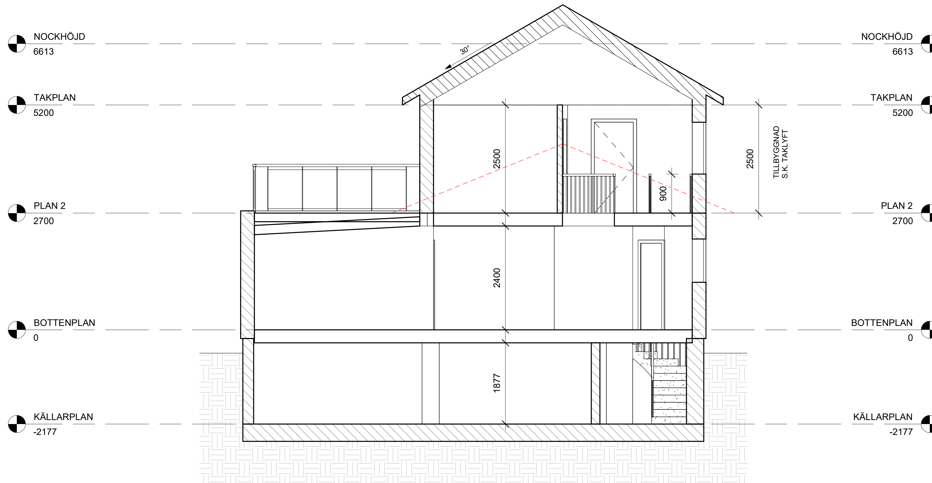
A SEKTION A-A 1 : 50
