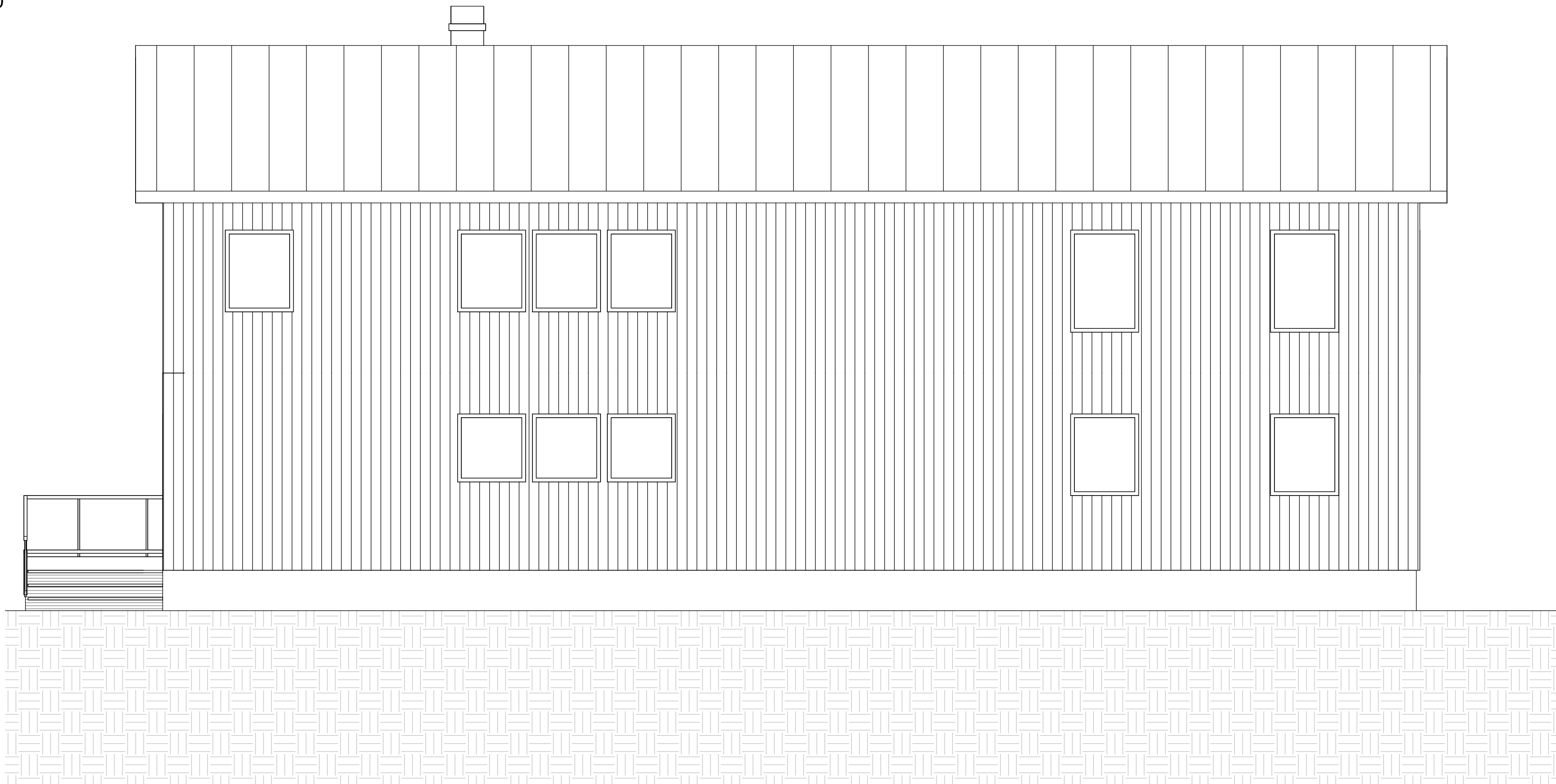
7 FASAD ÖSTER 1 : 50
