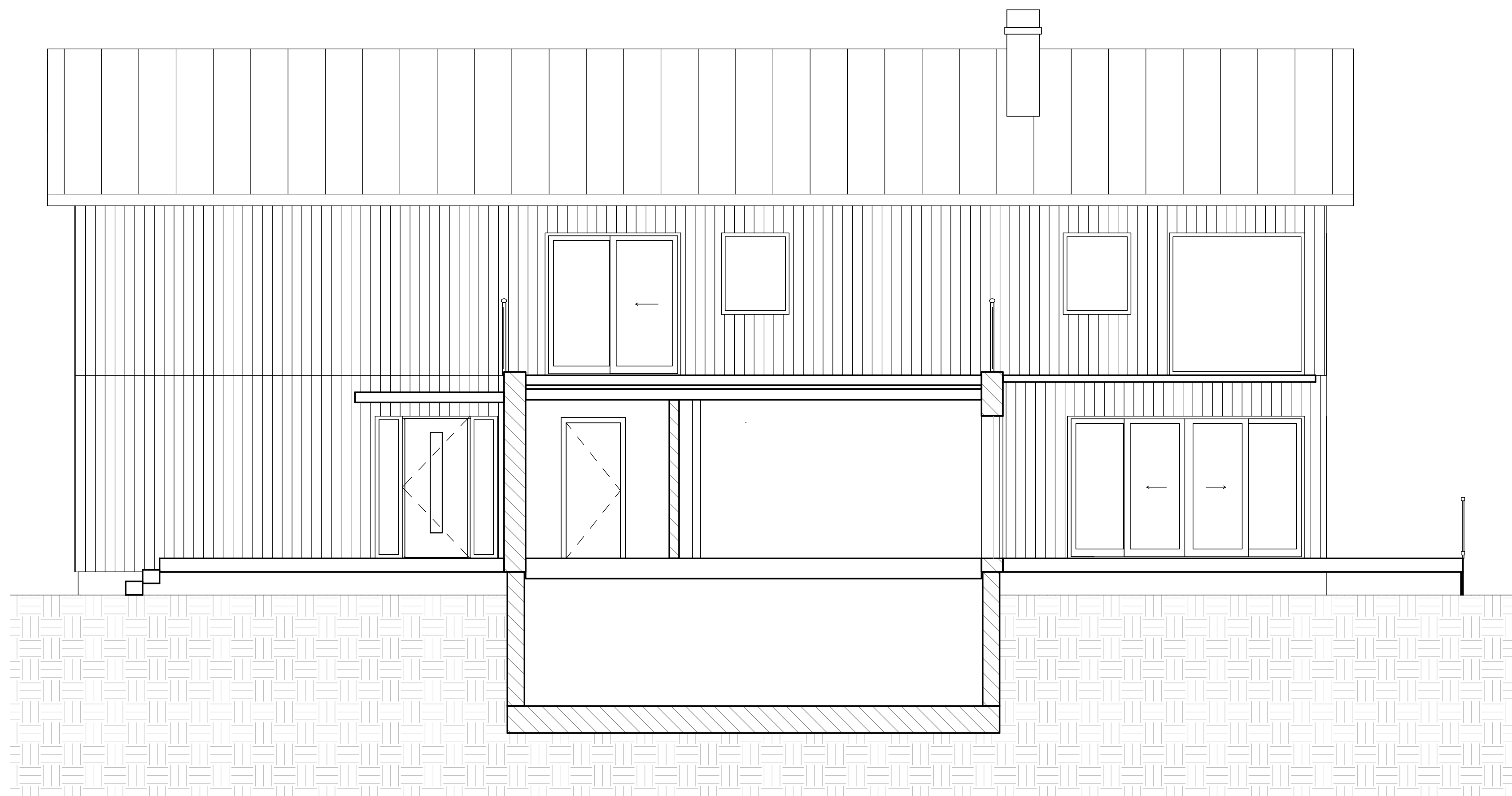
A SEKTION A-A 1 : 50
