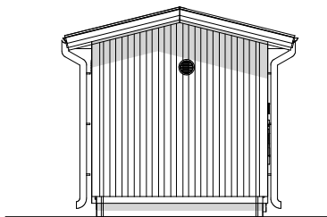
S1 FASAD MOT SÖDER
