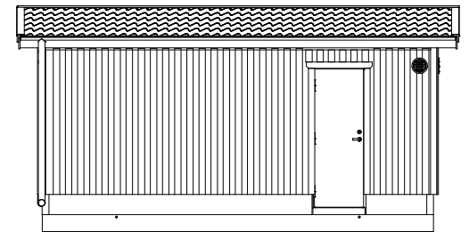
Fasad 3
