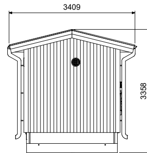
Fasad 4
