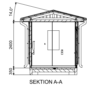
SEKTION A-A
